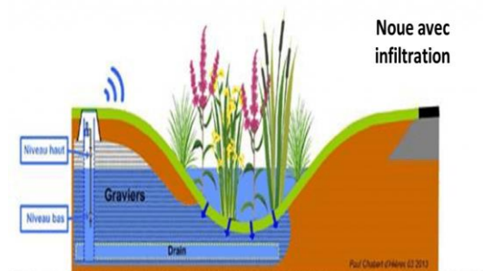
Figure 10 : Schéma d'une noue d'infiltration (source : site internet ADOPTA)
